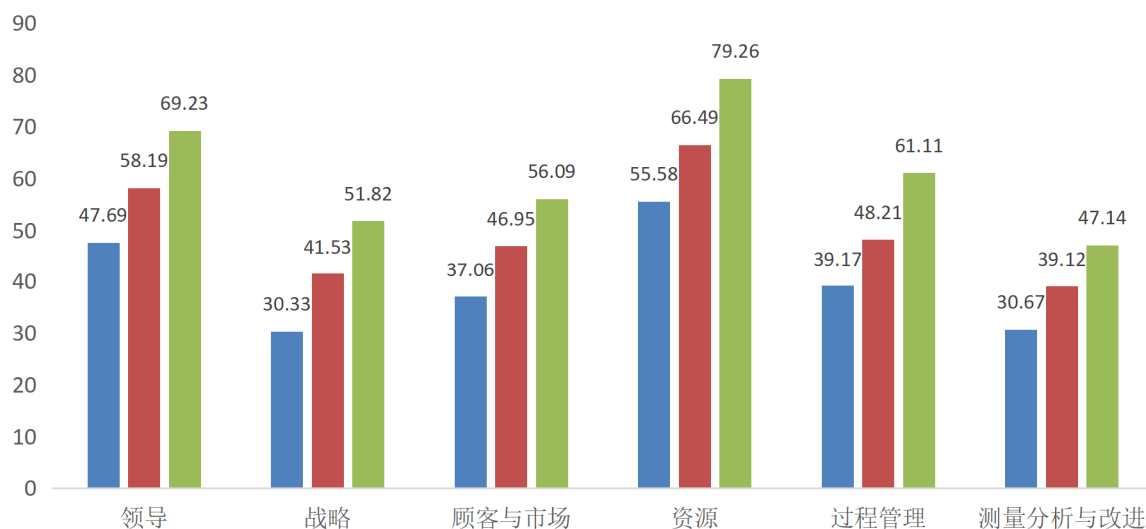
图 5-2 聚类结果六要素得分描述性统计图
